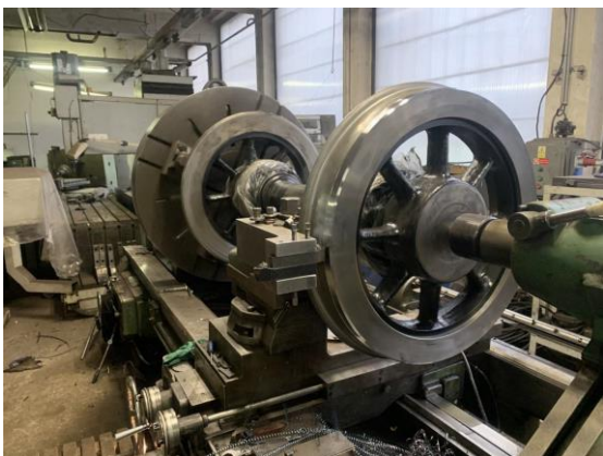
Soustružení profilu obručí běžných dvojkolí ve vlastní dílně zhotovitele
